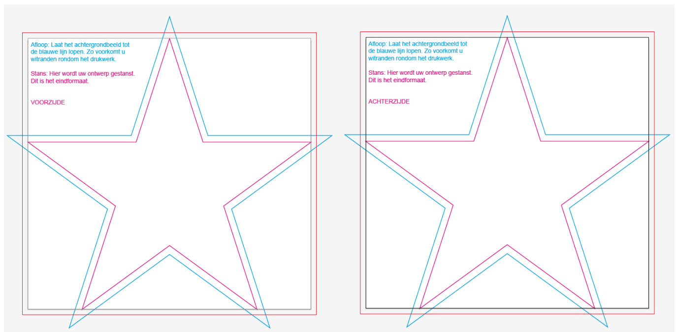
De voorzijde van de stans.
